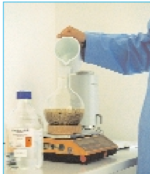
Destillation von Kamillenblüten zur Gewinnung des ätherischen Öls: Einwaage von Kamillenblüten und Wasser (links) sowie Aufbau der Destillations-Apparatur im Labor (rechts).
